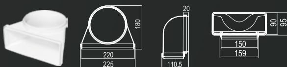
Horizontalni prehodni člen M2CKCF03U
