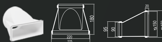
Vertikalni prehodni člen M2CKCF02U
