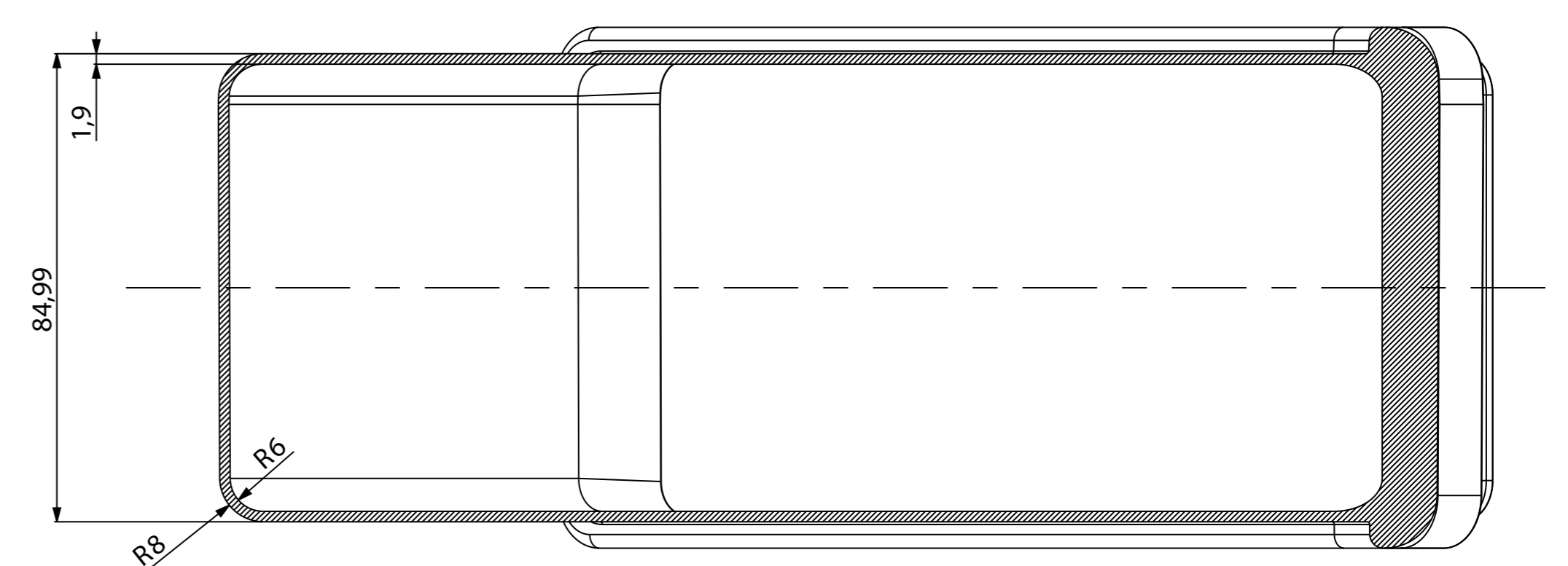
SEZIONE D-D
