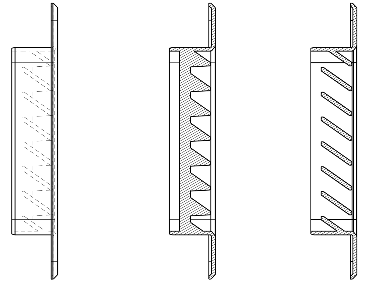
SEZIONE A-A
